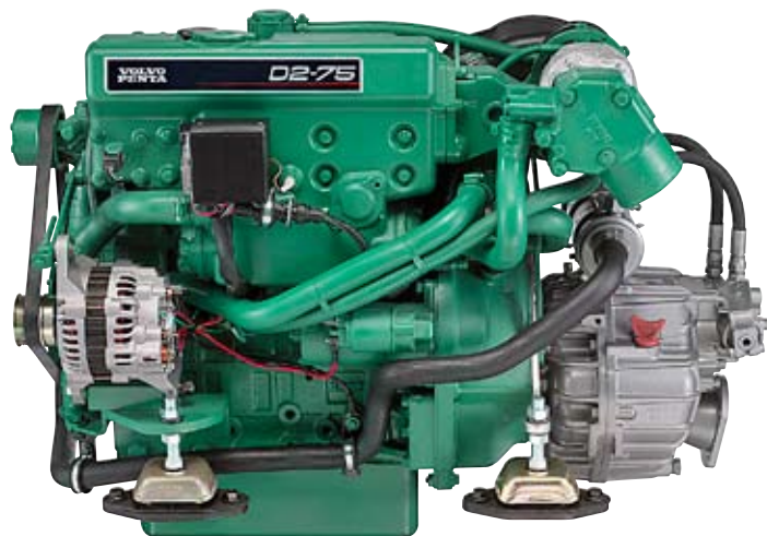
Volvo Penta D2-75 är en av det svenska företags moderna motorer, men inte ens till den rekommenderar företaget biodiesel. Den miljövänligare biodieseln kan bland annat härskna i filter och tankar.
